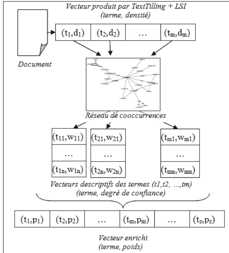
Figure 4 : Enrichissement des vecteurs de Termes
