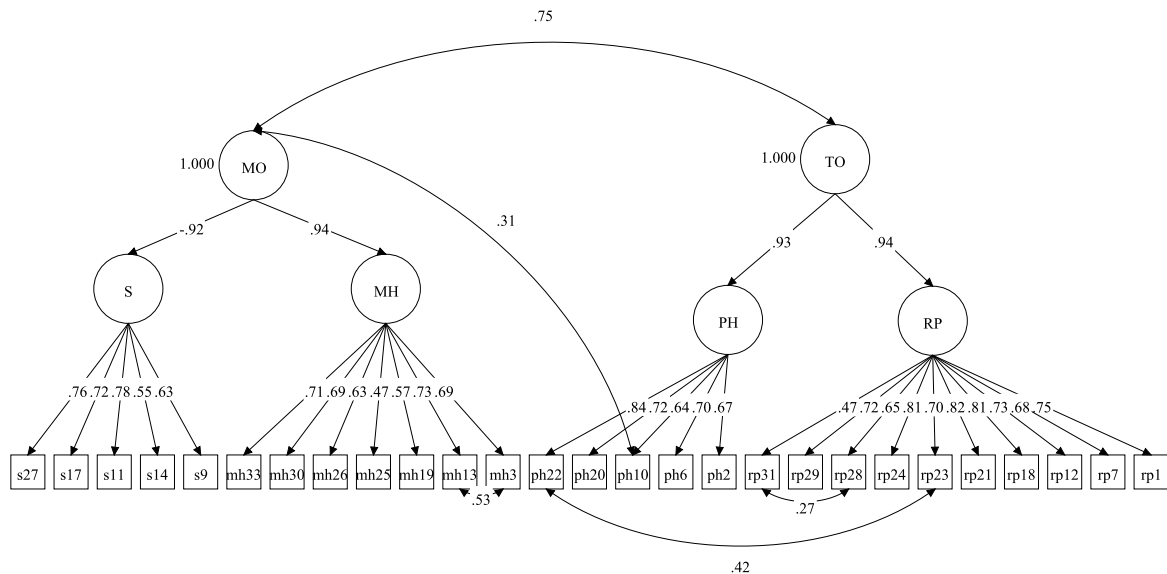
Figura 2 – Soluzione standardizzata del modello sottoposto ad analisi fattoriale confermativa della SMAVDLUG con fattori di secondo ordine ( N = 476 ).
