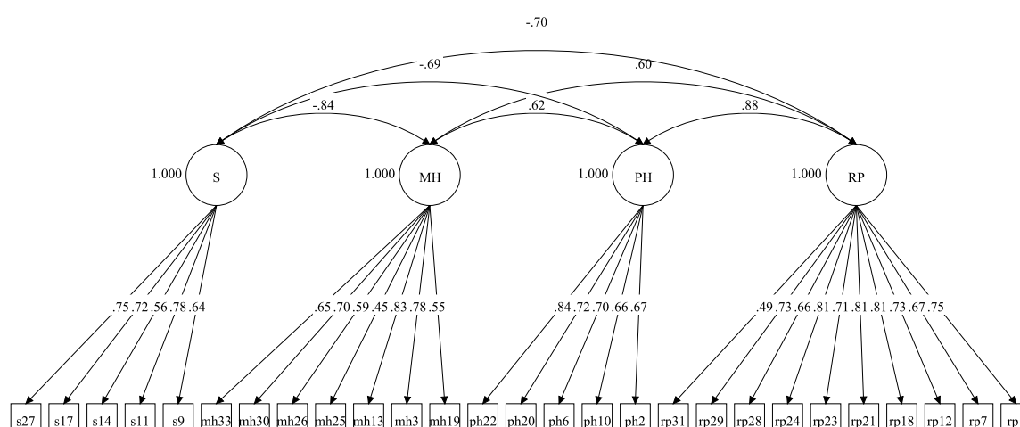
Figura 1 – Soluzione standardizzata del modello sottoposto ad analisi fattoriale confermativa della SMAVDLUG ( N = 476 )
