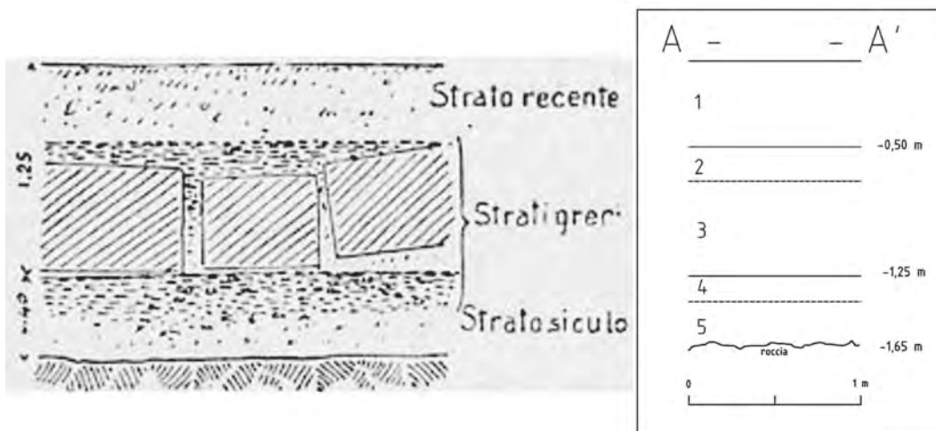
Fig. 6 – Siracusa, piazza Minerva: sezione A-A' e sua elaborazione grafica (a destra).
