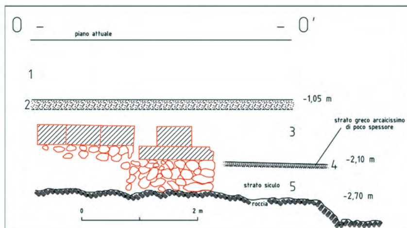
Fig. 41 - Siracusa, piazza Minerva: sezione O-O', disegno (in alto), e sua elaborazione grafica (in basso). Soprintendenza BB.CC.AA. di Siracusa, 1.19.2.231B.
