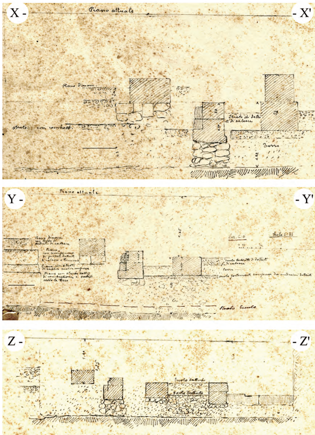
Fig. 54 – Siracusa, cortile del Palazzo Arcivescovile, dall'alto: sezioni X-X', Y-Y', Z-Z'. Soprintendenza BB.CC.AA. di Siracusa, 1.19.4.304B.
